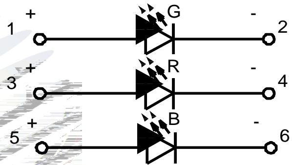
Fig.1-4 Polarity 极性
